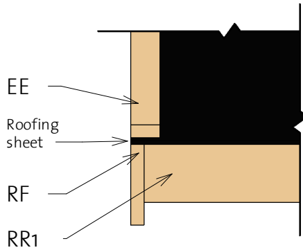
2) Facia
